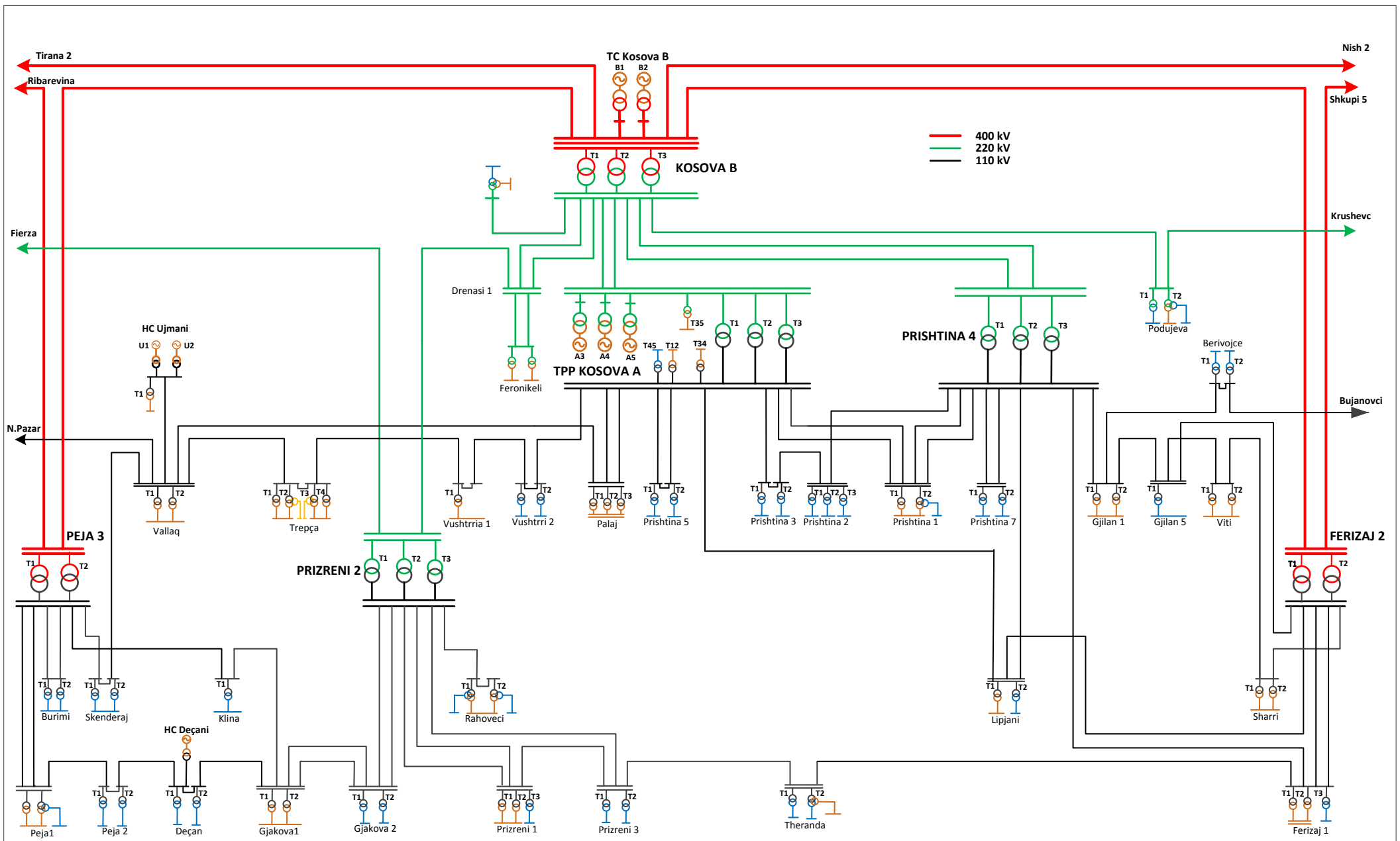
Skema njëpolare e SEE të Republikës së Kosovës - 2017
